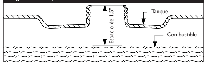
Figura 10 - Espacio de Combustible
